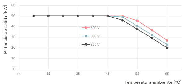
Reducción de potencia por sobre temperatura
