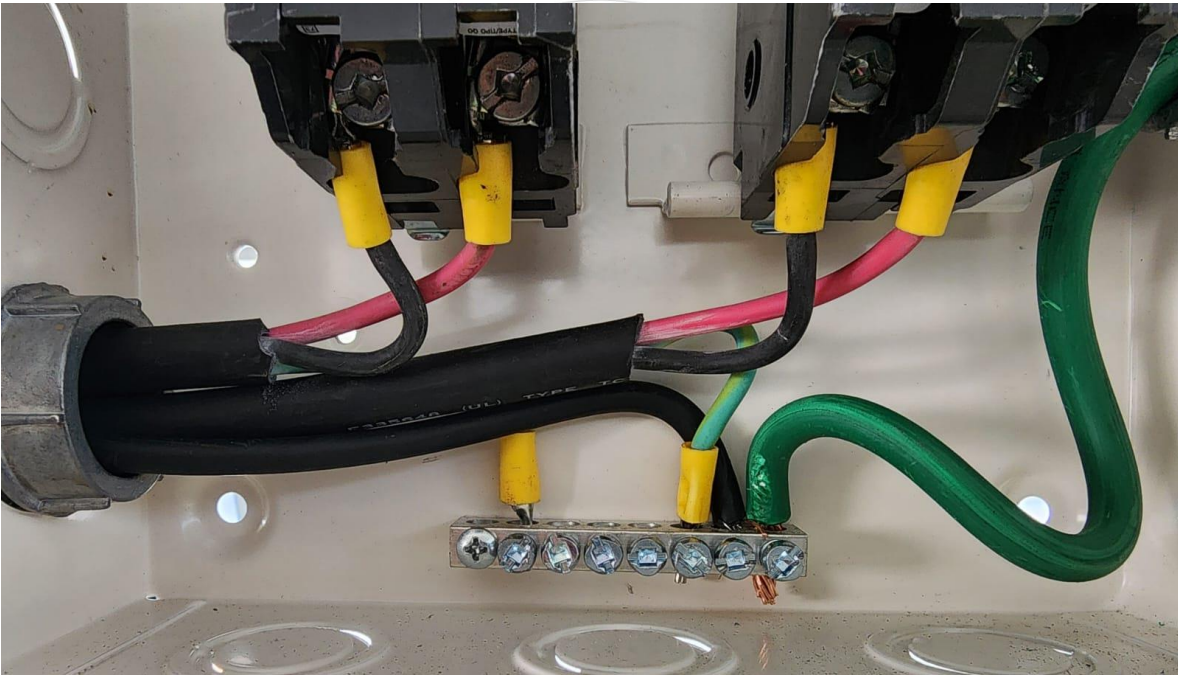
Conexión de protecciones CA.
